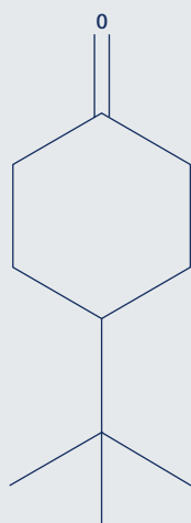
4-t-butylcyclohexanone
