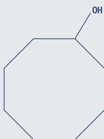
Cyclooctanol
